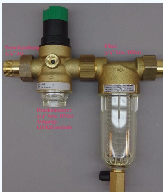
Abb. 7: Variante 2 – mit reduzierenden Verschraubungen auf 1/2"
