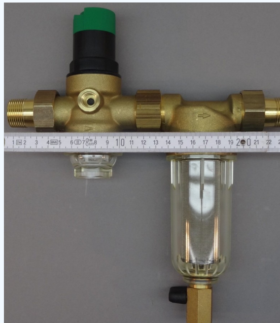
Abb. 5: Mit Linksgewinde am Ausgang – 24 cm, Platzersparnis 10 cm
