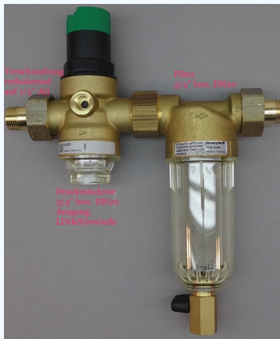
Abb. 6: Variante 1 – mit Verschraubungen in 3/4"
